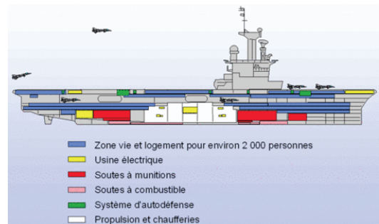
Coupe longitudinale du porte-avions
