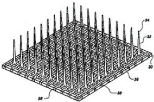
Grille d'électrodes « Utah »
